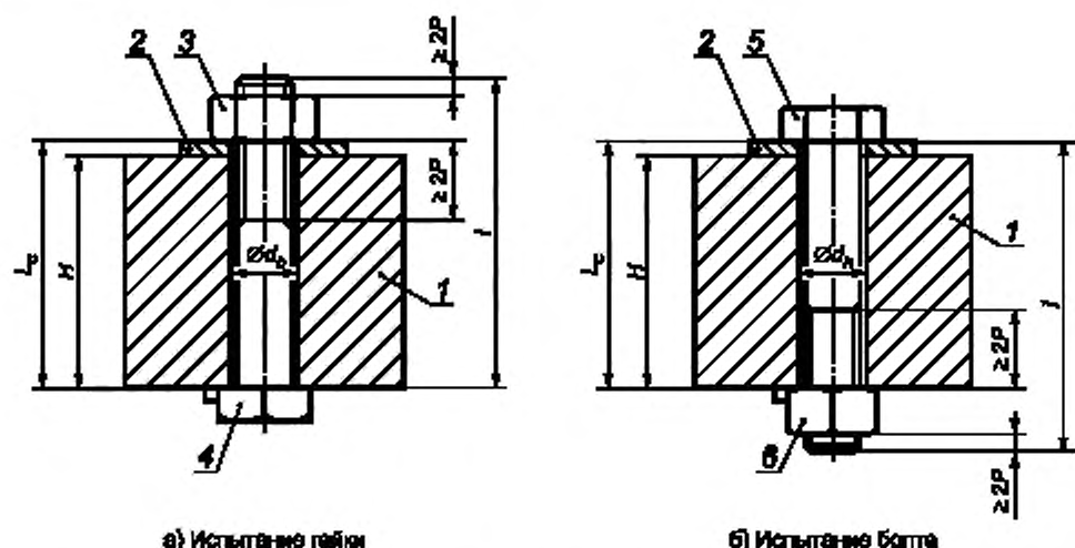
1 — приспособление для затяжки; 2 — опорная пластина; 3 — проверяемая гайка; 4 — сменный болт; 5 — проверяемый болт; 6 — сменная гайка
