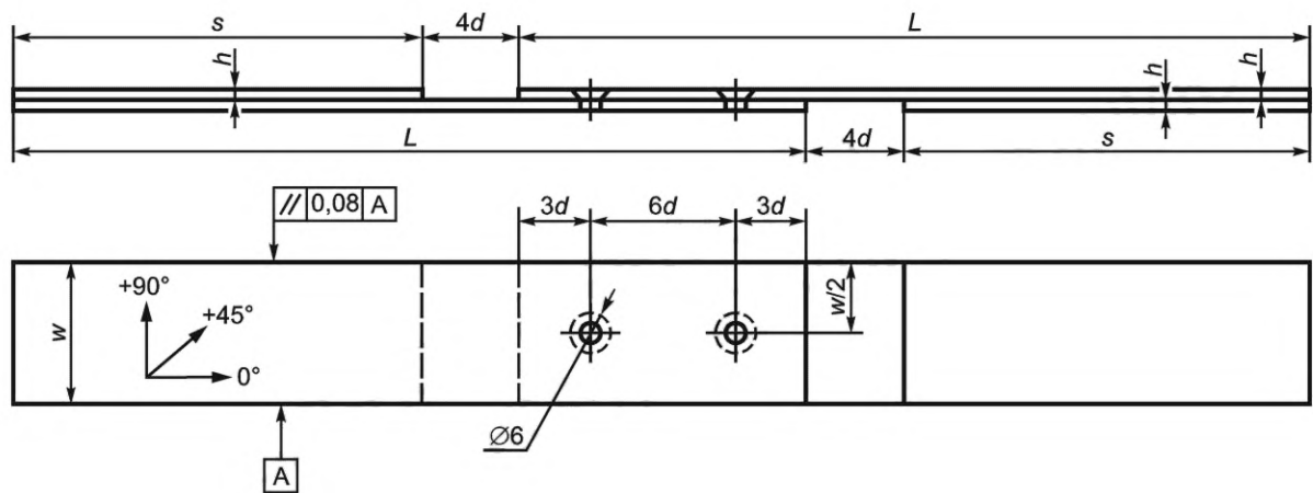
s — длина накладки; h — толщина полосы и накладки; L — длина полосы; w — ширина полосы; d — диаметр отверстия Рисунок 3 — Форма и размер составных образцов для испытаний по методу Б
