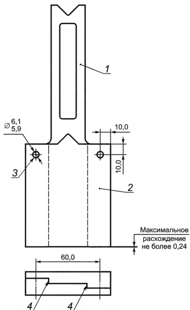
Рисунок Б.2 — Конструкция длинного зажима
