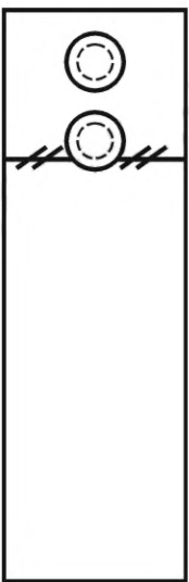
Рисунок В.14 — Разрушение при сжатии типа LGF: поперечное разрушение по краю крепления, гайки, шайбы (как правило происходит вдоль направления армирования 0°)
