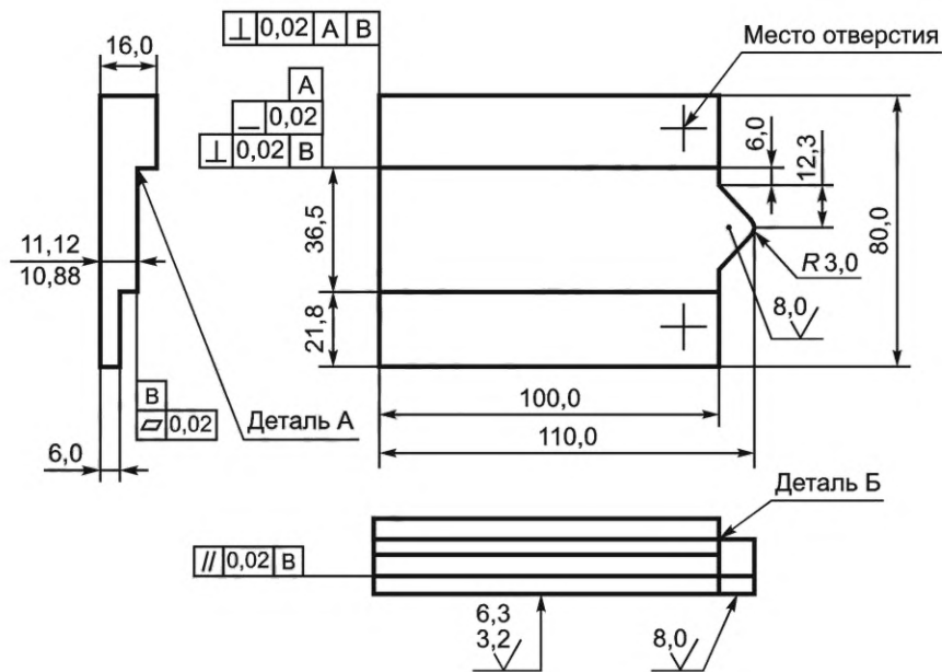
Рисунок Б.4 — Размеры короткого зажима
