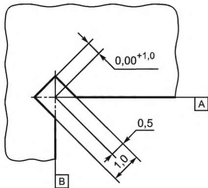
Рисунок Б.5 — Деталь А (размеры подреза)
