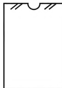
Рисунок В.6 — Разрушение при растяжении типа LGM: поперечный отрыв через центр отверстия (может сопровождаться расслаиванием и разделением на части)
