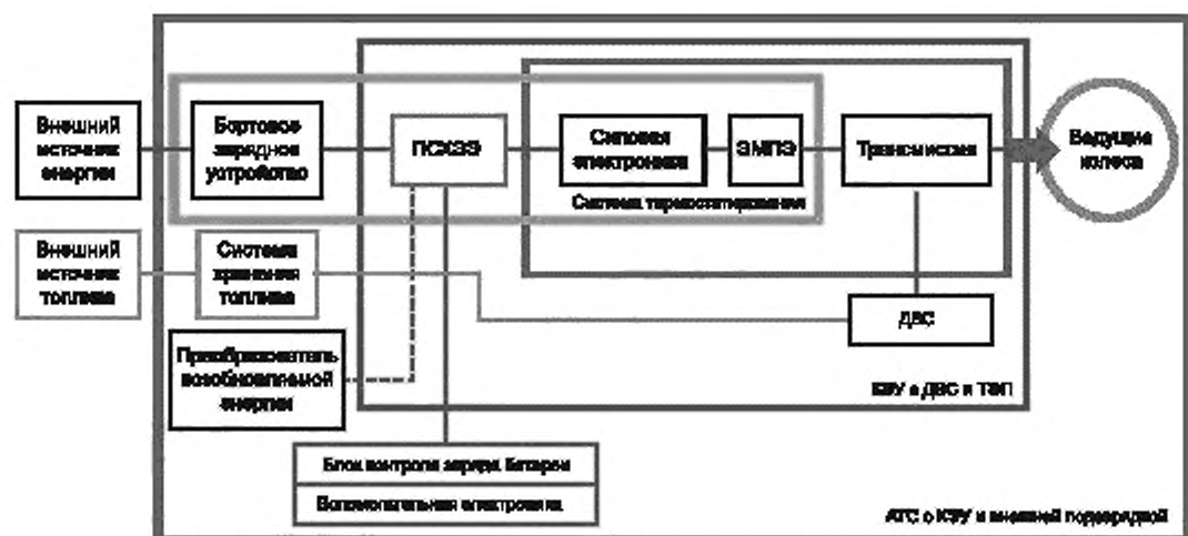
Рисунок А.3 — Возможная схема автомобильного транспортного средства с комбинированной энергоустановкой, имеющей возможность внешней зарядки
