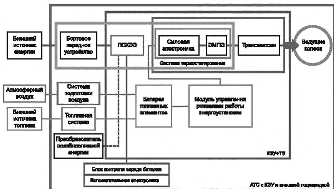
Рисунок А.4 — Возможная схема автомобильного транспортного средства с комбинированной энергоустановкой на топливных элементах
