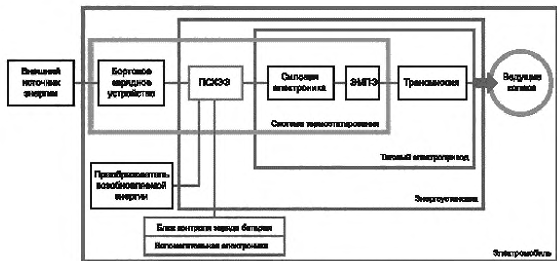
Рисунок А.1 — Возможная схема электромобиля
