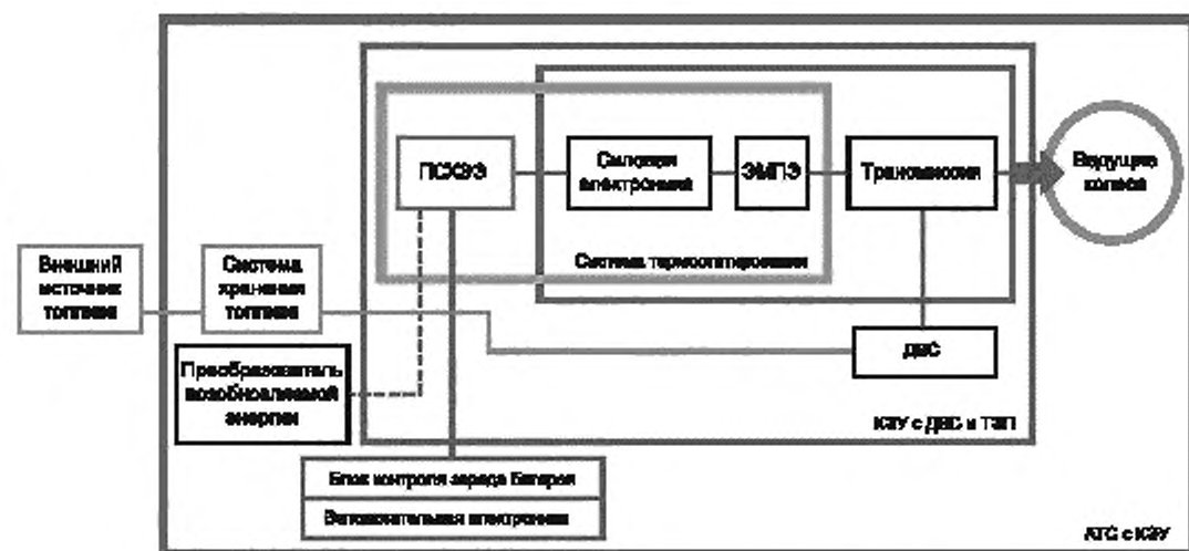
Рисунок А.2 — Возможная схема автомобильного транспортного средства с комбинированной энергоустановкой параллельного типа без возможности внешней зарядки
