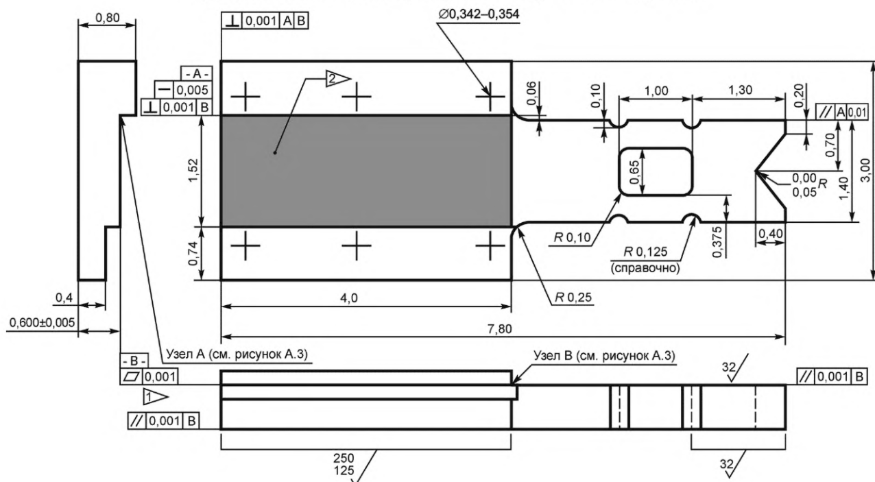
Рисунок А.1 — Размеры длинного захвата
