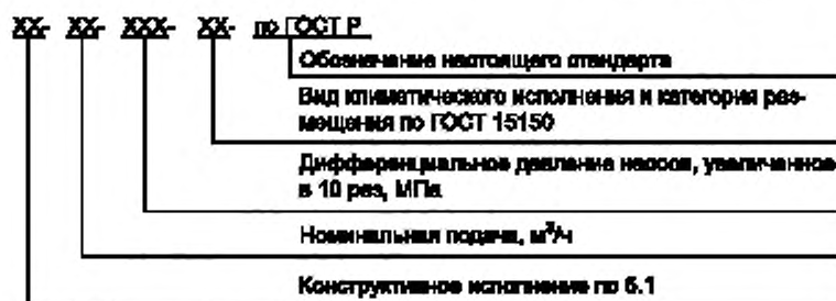
Рисунок 2 — Рекомендуемая схема условного обозначения винтового вертикального полупогружного насоса
