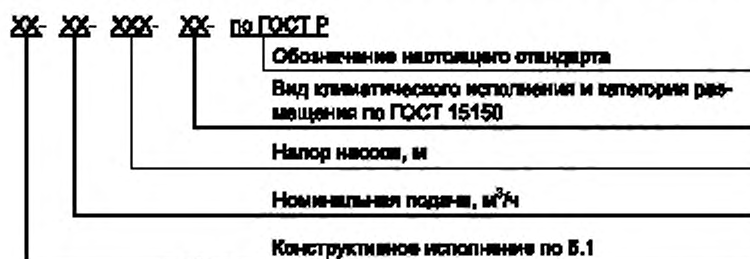
Рисунок 1 — Рекомендуемая схема условного обозначения центробежного вертикального полупогружного насоса
