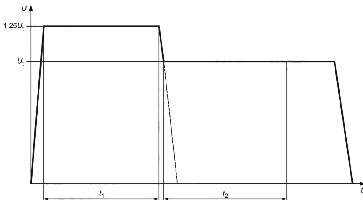
Рисунок 104 — Диаграмма зависимости испытательного напряжения от времени
