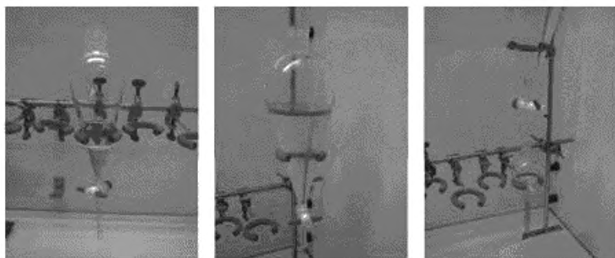
Рисунок В.3 — Порядок экстракции адсорбента Тепах® и сбора фазы петролейного эфира (см. 7.4.3)
