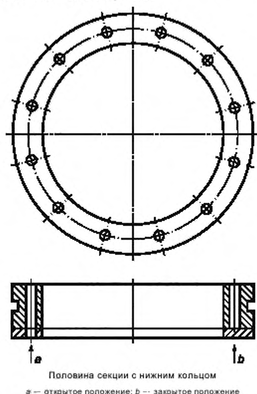
Рисунок А.1 — Схема типового регулируемого воротникового устройства
