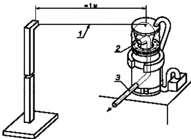
1 — эластичный шнур, обеспечивающий беспрепятственное перемещение капюшона в вертикальном направлении; 2 — регулируемое воротниковое устройство (см. рисунок А.1); 3 — концентрические трубки, присоединенные к дыхательной машине
