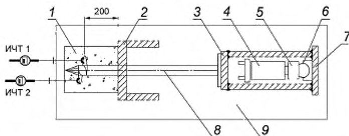
1 — обойма; 2 — жесткая заделка; 3 — фланец для передачи нагрузки; 4 — гидравлический домкрат; 5 — динамометр сжатия; 6 — шаровая опора; 7 — упорная стенка; 8 — свая; 9 — испытательный стенд; ИЧТ — индикатор часового типа
