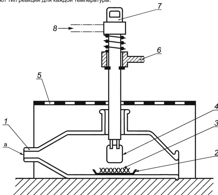
1 — стеклянный корпус; 2 — контейнер для образцов; 3 — испытуемый образец; 4 — нить накала (вольфрамовая нить); 5 — защитная решетка; 6 — фиксированная резьбовая опора; 7 — ручка; 8 — реостат; а — подача кислорода
