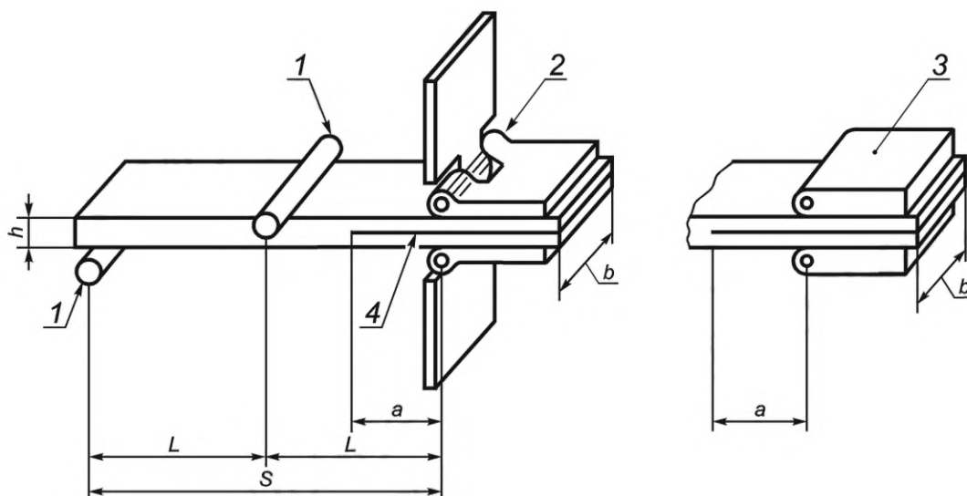
а) Оснстка для комбинированного нагружения образца
