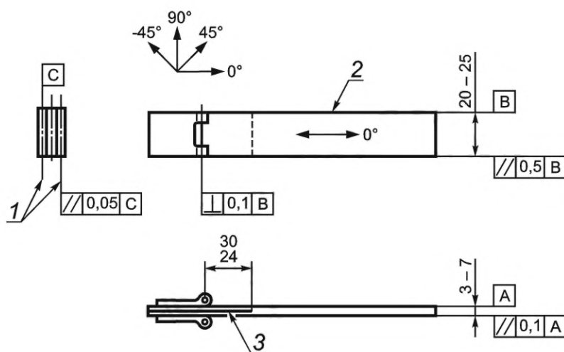
Рисунок 3 — Образец для испытания в условиях комбинированного нагружения отрывом и сдвигом
