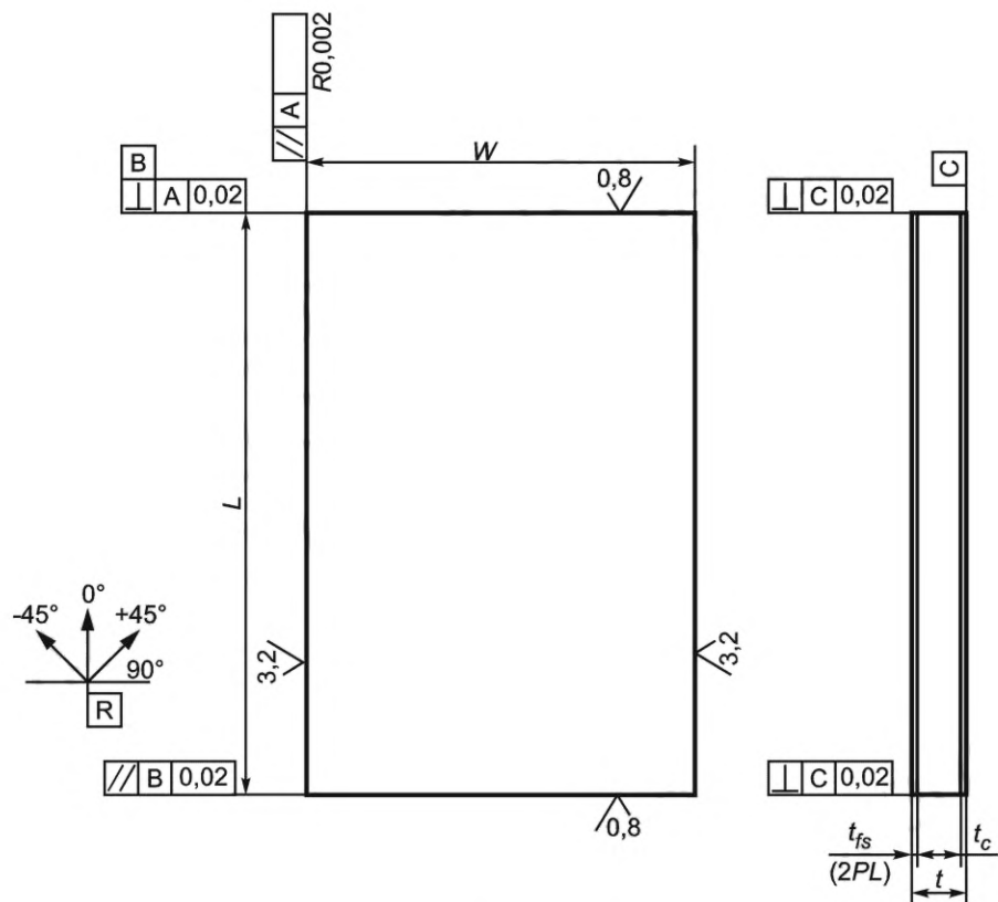
Рисунок 1 — Размеры образцов
