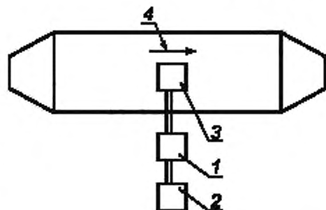
Рисунок 6 — Схема установки для процедуры В (в испытательной пылевой камере находится только место входа воздуха в СИЗОД)
