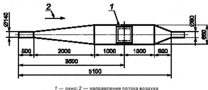
Рисунок 2 — Размеры рекомендуемой испытательной пылевой камеры
