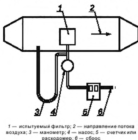
Рисунок 4 — Схема установки для методики А
