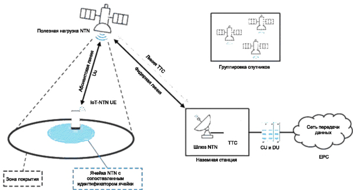
Рисунок 32 — Схема NTN-связи
