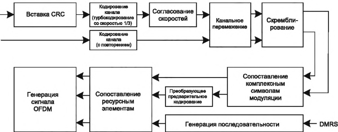
Рисунок 17 — Обработка физического uplink-канала
