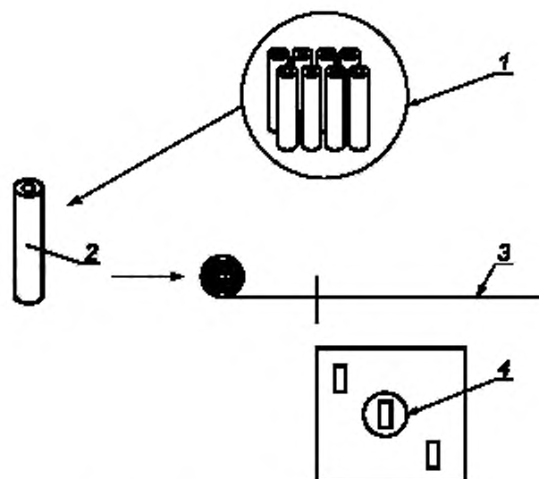
1 — партия; 2 — выборка; 3 — полоса материала; 4 — образцы для испытаний
