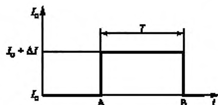
Рисунок 9 — Проверка реакции регулятора тока инвертора на входное ступенчатое воздействие
