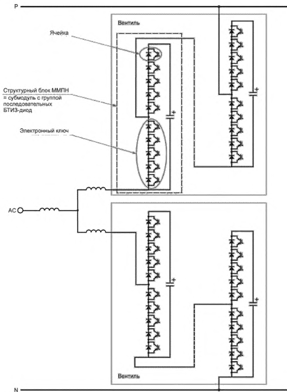
Рисунок 5 — Фазный блок каскадного двухуровневого преобразователя напряжения на основе submodule с группой последовательных ППЗ-диод
