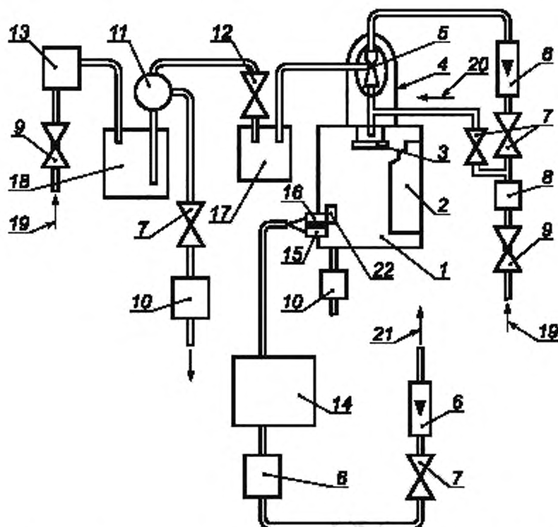
1 — испытательная камера; 2 — герметично закрываемая дверь камеры; 3 — тарелка для сбора масла, стекающего вниз по стенкам трубки; 4 — крышка воздуходувок, приводимых в движение напором воздуха; 5 — воздуходувки, приводимые в движение напором воздуха; 6 — расходомеры, действующие в диапазоне измерения от 800 до 8000 \text{дм}^3/\text{мин} для измерения потока воздуха, приводящего в движение вентиляторы (5000 \text{дм}^3/\text{мин} ); 7 — клапаны, регулирующие расход потока; 8 — высокоэффективные фильтры; 9 — регулятор подачи сжатого воздуха; 10 — высокопроизводительный воздушный фильтр; 11 — тройник для отбора аэрозоля парафинового масла, необходимого для испытания; 12 — игольчатый клапан, регулирующий концентрацию аэрозоля парафинового масла в камере; 13 — генератор аэрозоля парафинового масла; 14 — аэрозольный фотометр; 15 — пробоотборник для измерения концентрации аэрозоля парафинового масла в камере; 16 — пробоотборник для измерения концентрации аэрозоля парафинового масла после фильтра; 17 — склянка Вульфа; 18 — объем буфера 5 \text{дм}^3 ; 19 — сжатый воздух; 20 — подача воздуха для разбавления; 21 — к вакуумному насосу; 22 — испытуемый образец
