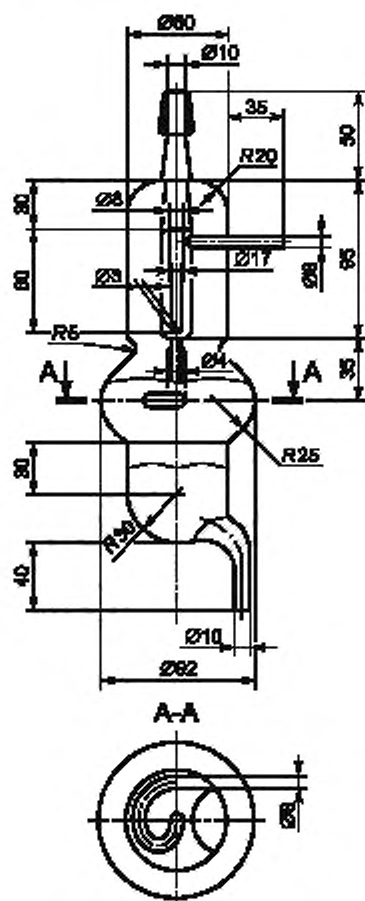
Рисунок 5 — Циклон
