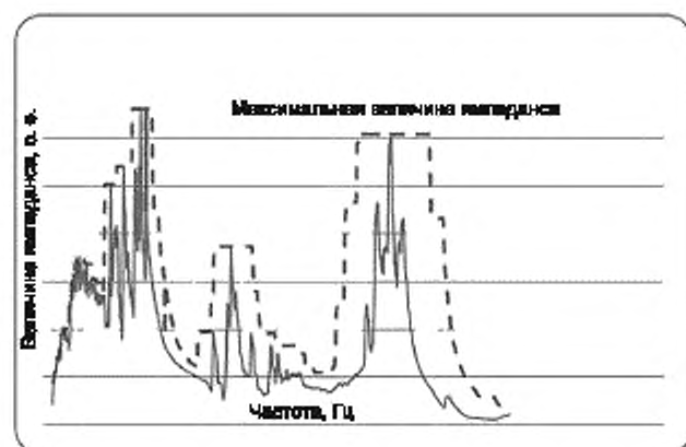
Рисунок 10 — Применение диапазона допусков в процентах номера гармоники
