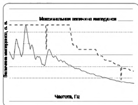
Рисунок 11 — Применение диапазона допусков в процентах номера гармоники, подынтервал, демонстрирующий 11-ю и 13-ю гармоники
