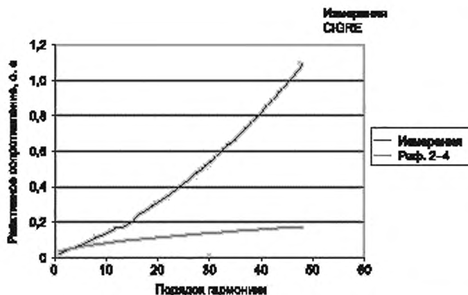
Рисунок Б.7 — Сравнение активного сопротивления синхронной машины с точки зрения рекомендаций CIGRE и испытаний явнотолкового генератора 370 МВА
