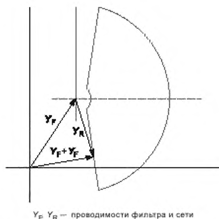
Рисунок Д.2 — Геометрическое представление выбора сопротивления при наихудших условиях для гармоник преобразователя
