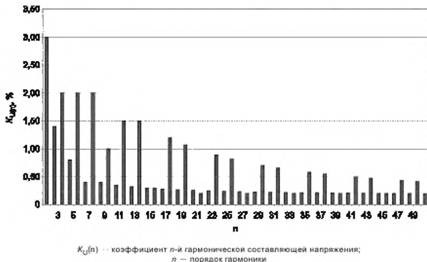
Рисунок Е.3 — Допустимые уровни МЭК, используемые для напряжений источников в исследовании
