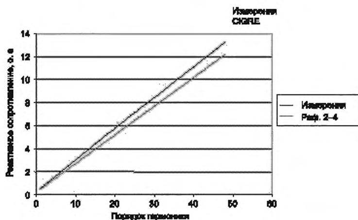
Рисунок Б.6 — Сравнение реактивного сопротивления синхронной машины с точки зрения рекомендаций CIGRE и испытаний явнополюсного генератора 370 МВА
