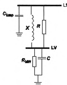
L1 — шина питания, LV — шина нагрузки низкого напряжения; C_{\text{ump}} — сосредоточенная емкость; X — сосредоточенное реактивное сопротивление трансформатора; R — демпфирующее сопротивление; R_{\text{MW}} — активная резистивная нагрузка; C — емкость низкого напряжения
