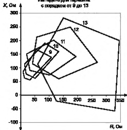
Импеданс для гармоник с порядком от 9 до 13
