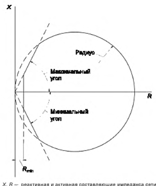
Рисунок Д.3 — Общая круговая диаграмма импеданса системы переменного тока, с минимальным активным сопротивлением R_{\min}
