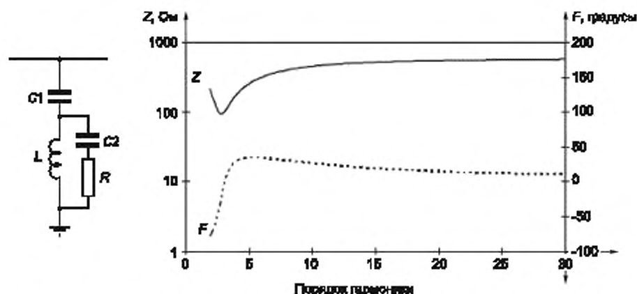
Рисунок В.5 — Широкополосный фильтр третьего порядка, амплитудно-частотная характеристика ( Z ), фазо-частотная характеристика ( F )
