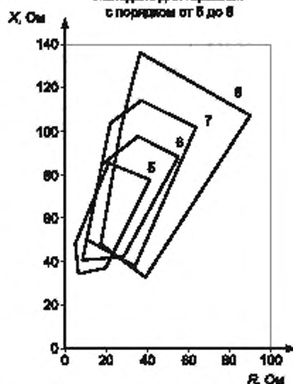
Импеданс для гармоник с порядком от 5 до 8
