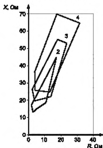
Импеданс для гармоник с порядком от 2 до 4
