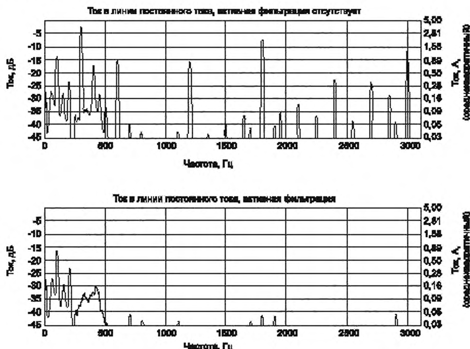
Рисунок Б.1 — Спектр измеренного тока в линии (полюс 3 работает как монополь)
