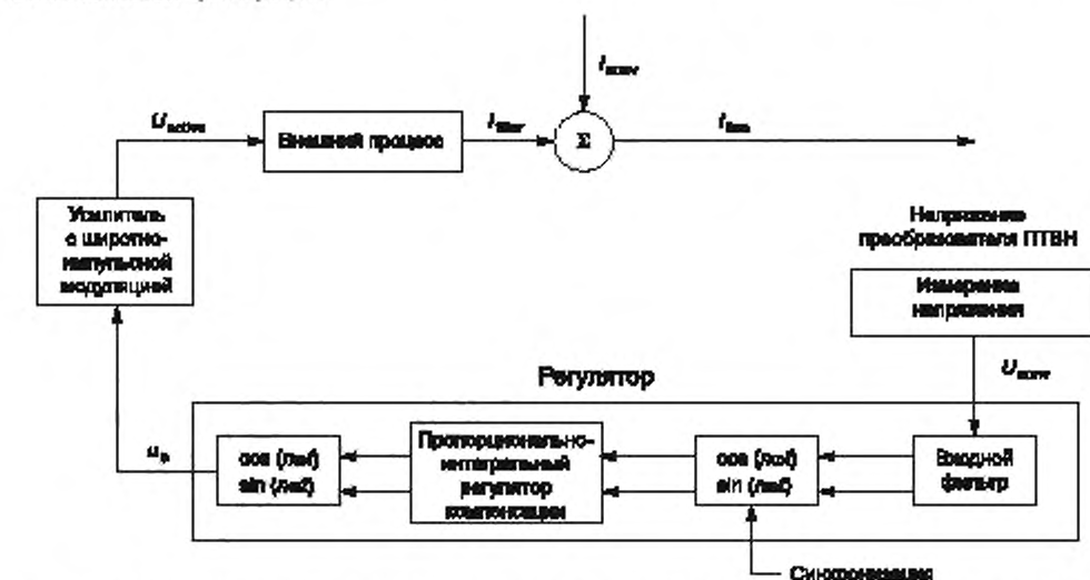
Рисунок 7 — Структурная схема системы управления активным фильтром с прямой связью
