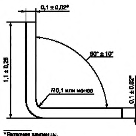
Рисунок 1 — Форма и размеры никелевой частицы
