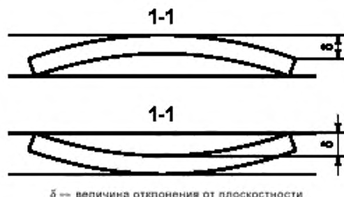
Рисунок 4 — Схема проверки АКЛ на отклонение от плоскостности
