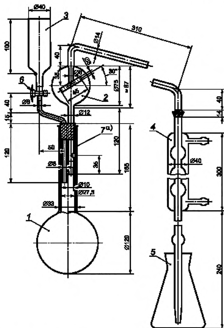
1 — круглодонная колба с длинным горлышком вместимостью 1000 см 3 , 2 — дистилляционная трубка с насадкой, предохраняющей от переброса перегоняемой жидкости, соединенная с холодильником с помощью шарового соединения (№ 18) (шаровое соединение с холодильником может быть заменено соответствующим резиновым соединением); 3 — воронка с политетрафторэтиленовым (PTFE) вентилем (6) для добавления гидроксида натрия (вентиль также может быть заменен резиновым соединением с зажимом); 4 — холодильник (шесть шаров) с шаровым соединением (№ 18) на входе, соединенный на выходе со стеклянной удлинительной трубкой с помощью небольшого резинового соединения (если присоединение дистилляционной трубки осуществляется с помощью резиновой трубки, шаровое соединение может быть заменено подходящей резиновой пробкой). 5 — колба для сбора дистиллята вместимостью 500 см 3 , 6 — вентиль из политетрафторэтилена (PTFE)
