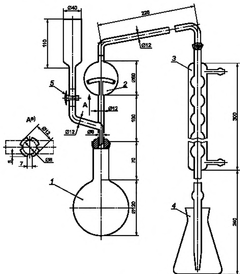
1 — круглодонная колба с коротким горлышком вместимостью 1000 см 3 с шаровым соединением (№ 35); 2 — дистилляционная трубка с насадкой, предохраняющей от переброса перегоняемой жидкости, с шаровым соединением (№ 35) на входе и шаровым соединением (№ 18) на выходе, соединенная сбоку с воронкой политетрафторэтиленовым (PTFE) вентилем (5) для добавления гидроксида натрия; 3 — холодильник (шесть шаров) с шаровым соединением (№ 18) на входе, соединенный на выходе со стеклянной удлинительной трубкой с помощью небольшого резинового соединения; 4 — колба для сбора дистиллята вместимостью 500 см 3 ; 5 — вентиль из политетрафторэтилена (PTFE)
