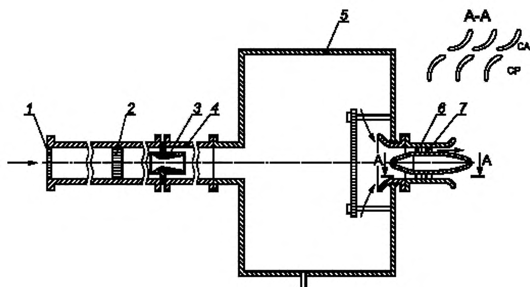
1 — сетка, 2 — секция струеуправляющей (хонейкомб); 3 — мерный участок; 4 — участок для измерения расхода газа; 5 — ресивер, 6 — СА; 7 — CP
