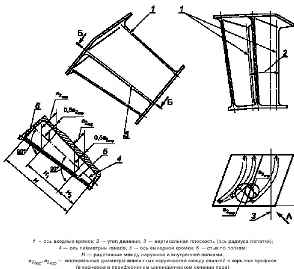
Рисунок 2 — Схема межлопаточного канала
