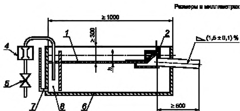
а) Парапетная воронка горизонтальная
