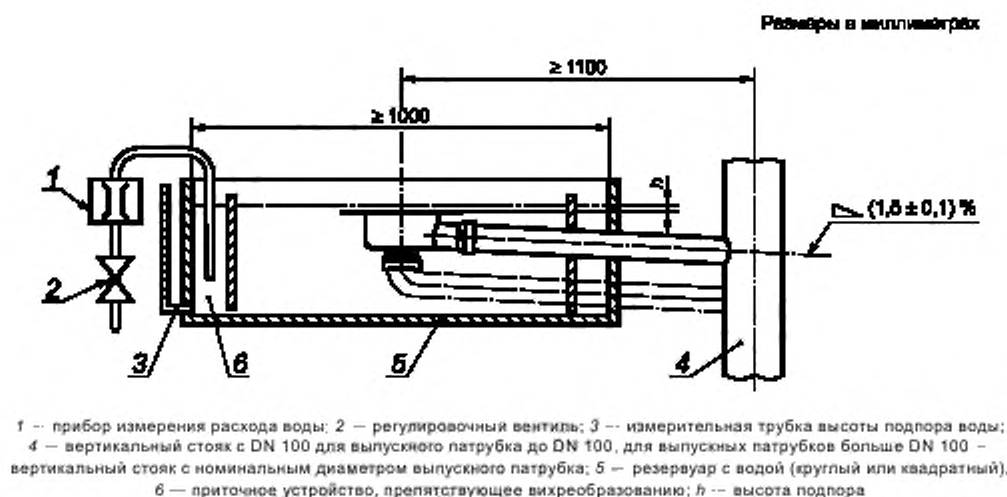
Рисунок 9 — Схема испытания для измерения пропускной способности водосточных трапов
