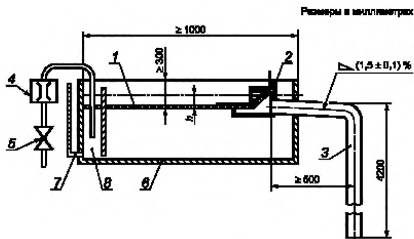
б) Парапетная воронка вертикальная
