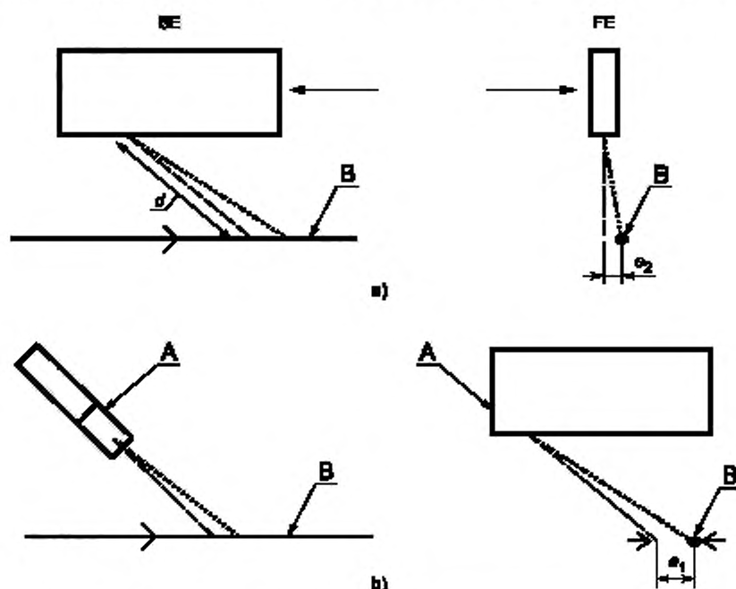
А — датчик; В — струна; SE — вид сбоку; FE — вид спереди; — — — — номинальное направление оси доплеровского пучка; ····· — действительное направление оси доплеровского пучка
