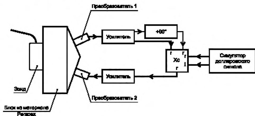
а) Электронный тест-объект
