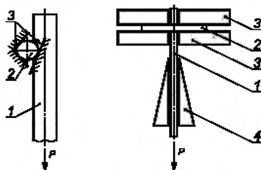
1, 2 — стержни; 3 — заделка стержня в приспособлении, 4 — захваты испытательной машины, P — испытательная нагрузка
