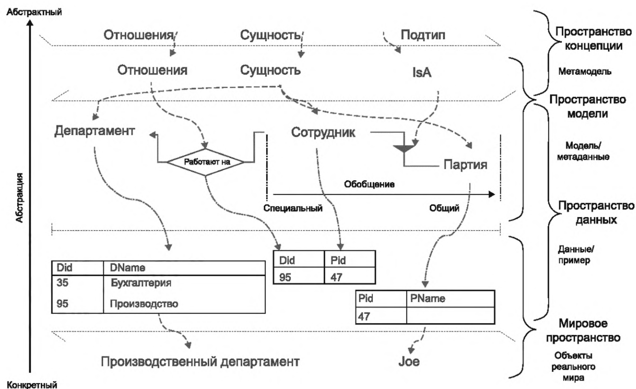
Рисунок 1 — Абстракции метаотношений
