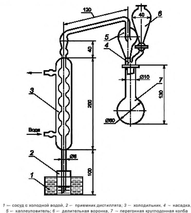
Рисунок А.1 — Установка для отгонки мышьяка
