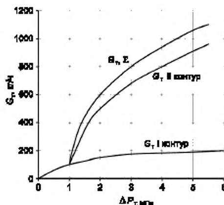
Рисунок Г.1 — Зависимость расхода топлива G_T через центробежную одноконтурную одноорословую форсунку от избыточного давления подачи топлива \Delta P_T ( T_T = 280 K)
