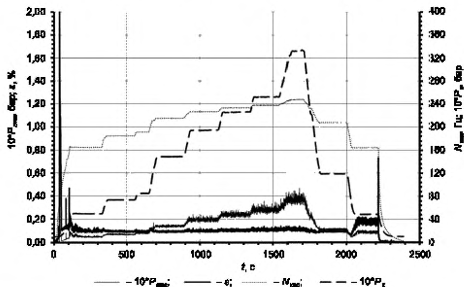
Рисунок Е.1 — Изменение частоты вращения КВД ( N_{ввд} ), полного давления воздуха на входе в КС ( 10P_{свз} ), относительного ( \epsilon = P_{rms}/P_{свз} ) и среднеквадратичного значения ( 10P_{rms} ) колебаний давления газа в зависимости от времени выхода газогенератора на заданные режимы работы
