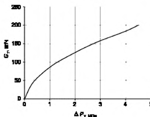
Рисунок Г.1 — Зависимость расхода топлива G_T через центробежную одноконтурную одноорословую форсунку от избыточного давления подачи топлива \Delta P_T ( T_T = 280 K)
