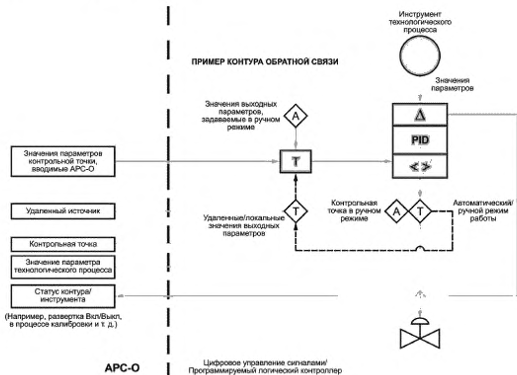
Рисунок 12 — Взаимодействие APC-О с исполнительным звеном (элементом) системы управления
