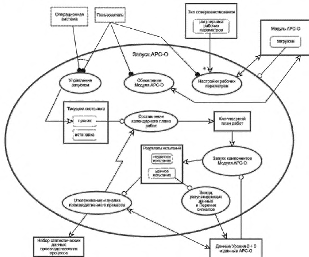
Рисунок 3 — Рабочий процесс стадии «исполнение»
