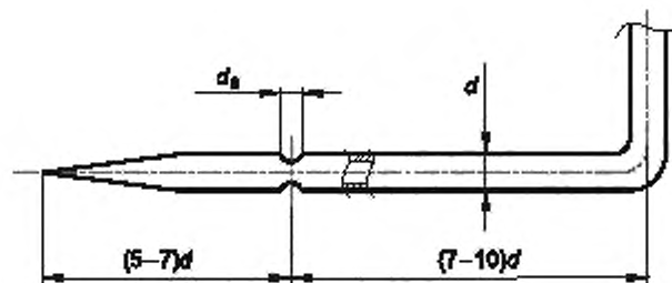
Рисунок 2 — Схема иглы-приемника статического давления
