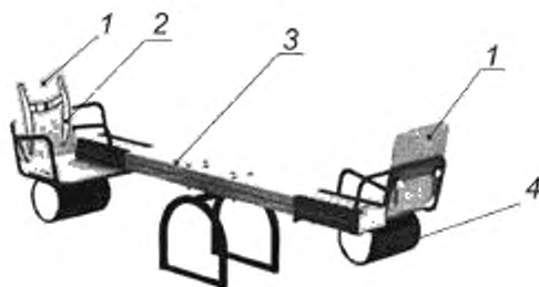
1 — сиденье; 2 — ремни безопасности; 3 — баланси́р; 4 — демпфер
