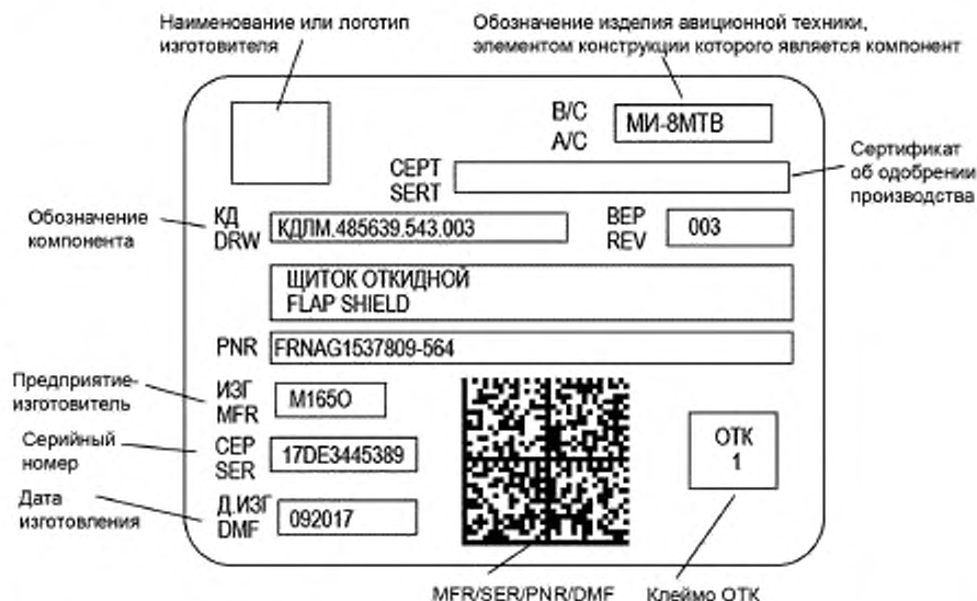
Рисунок 1 — Опознавательная табличка с полным составом данных по [1] для компонента АТ II класса, поле «PNR» на основной табличке в одном символе штрихового кода с данными MFR, SER, DMF
