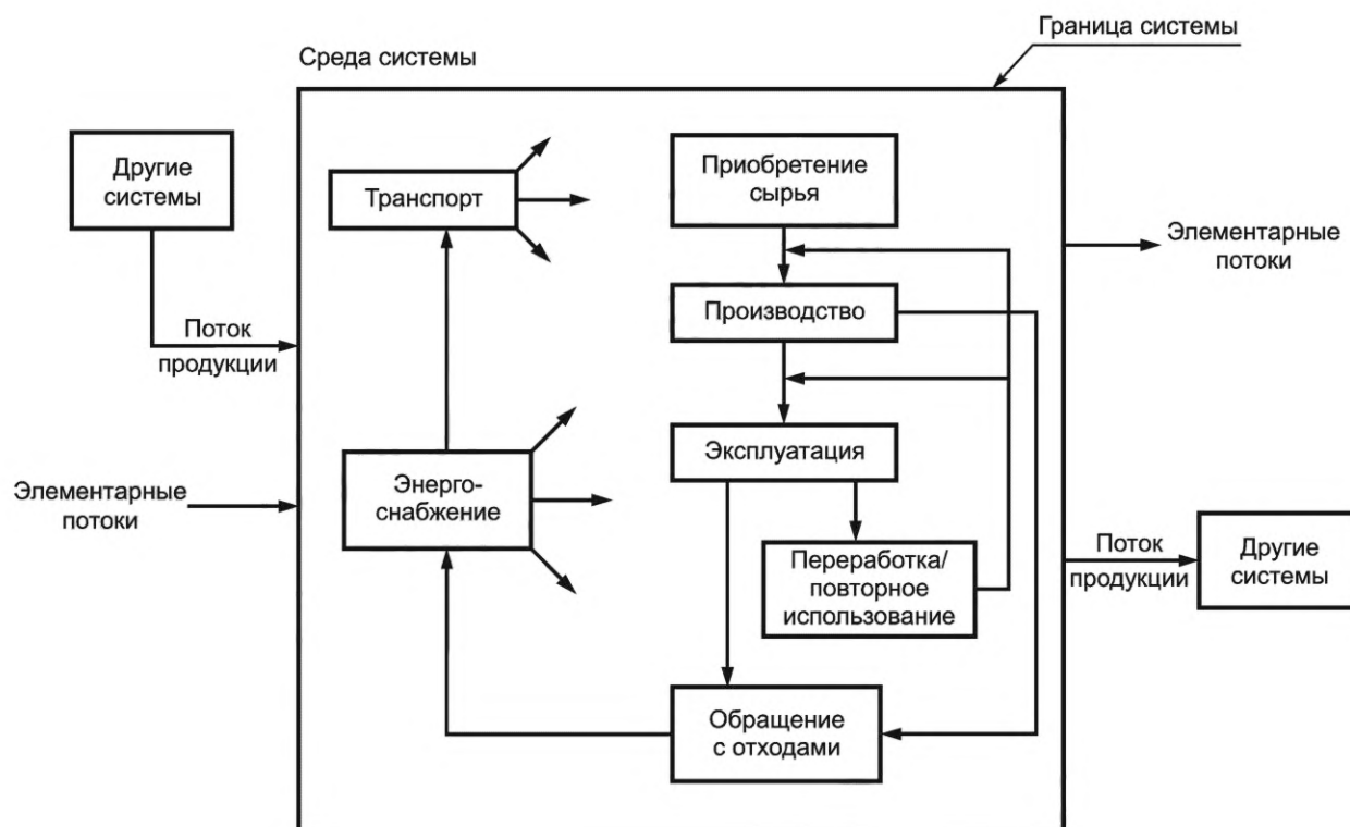
Рисунок 2 — Пример производственной системы для ОЖЦ
