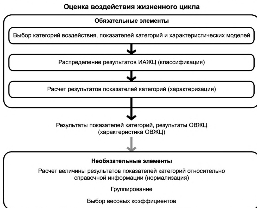
Рисунок 4 — Элементы стадии ОВЖЦ (характеристических моделей)
