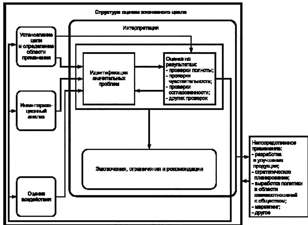
Рисунок 4 — Связь между элементами стадии интерпретации и другими стадиями оценки воздействия жизненного цикла
