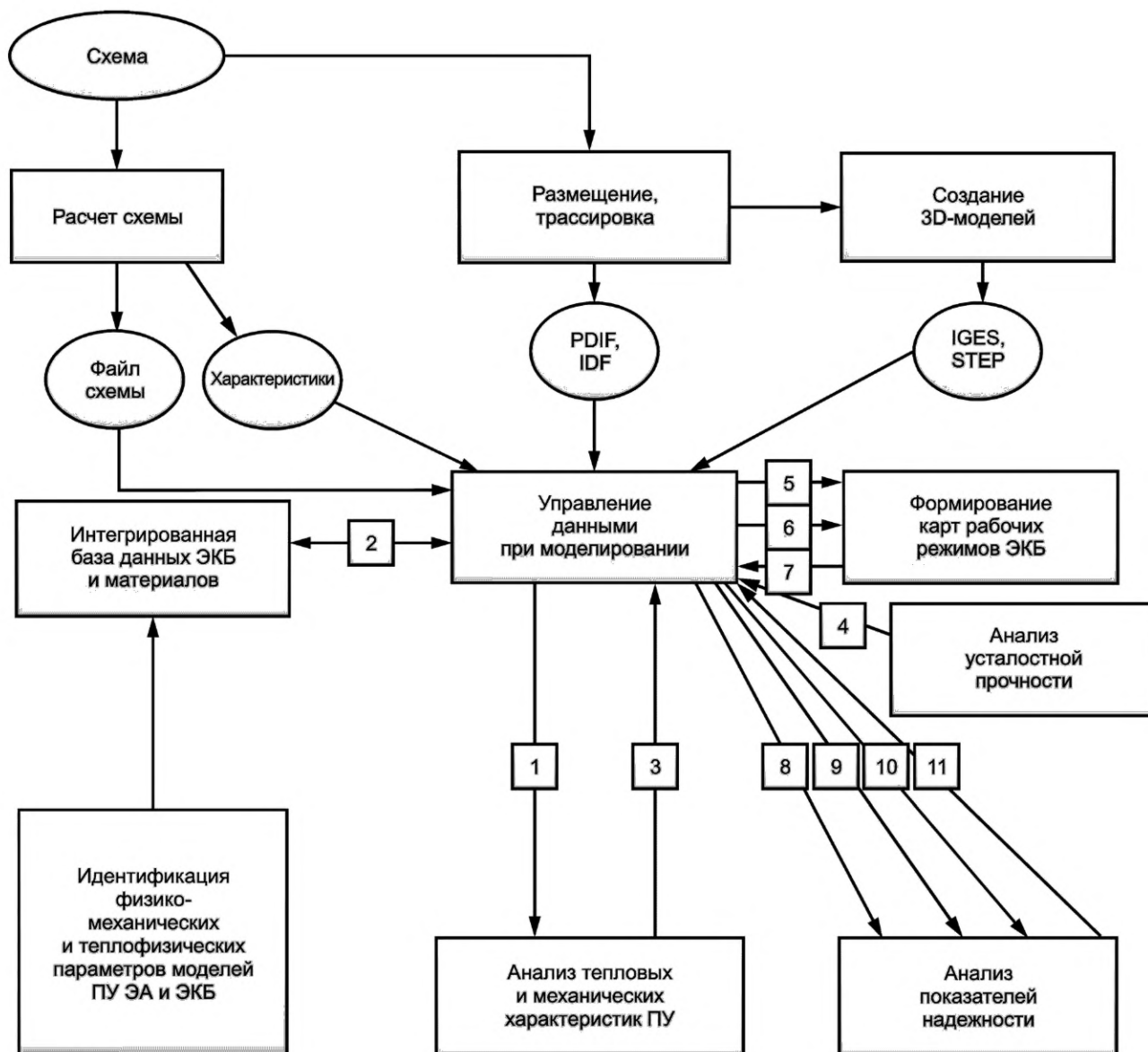
Рисунок 5.1 — Структурная схема САПР ПУ ЭА
