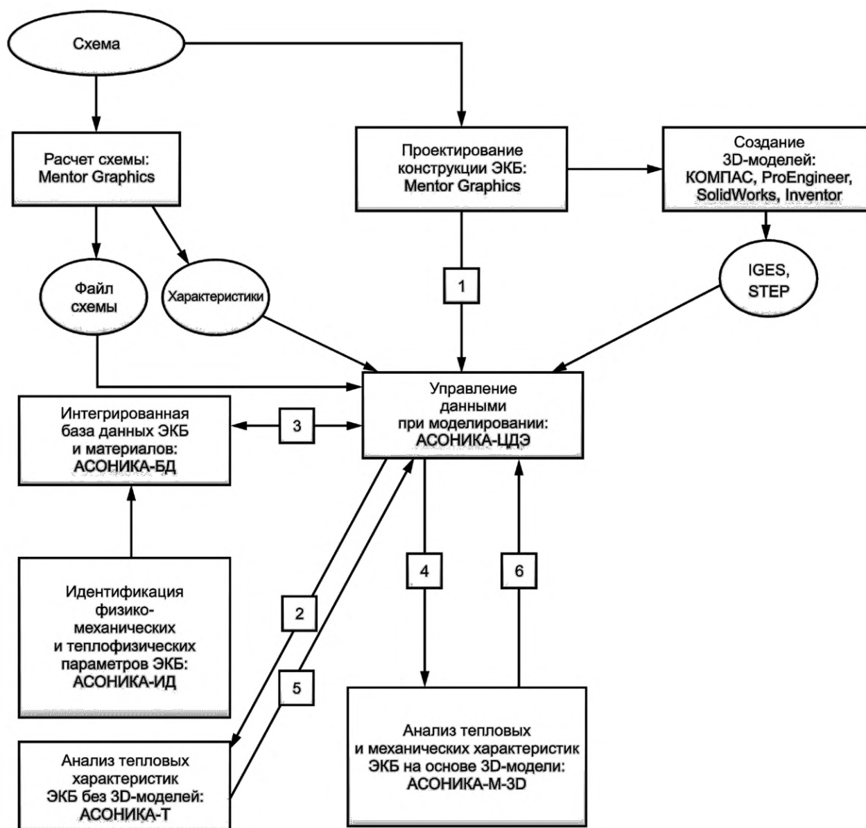
Рисунок А.1 — Структурная схема САПР ЭКБ, построенная на базе российской автоматизированной системы обеспечения надежности и качества аппаратуры АСОНИКА
