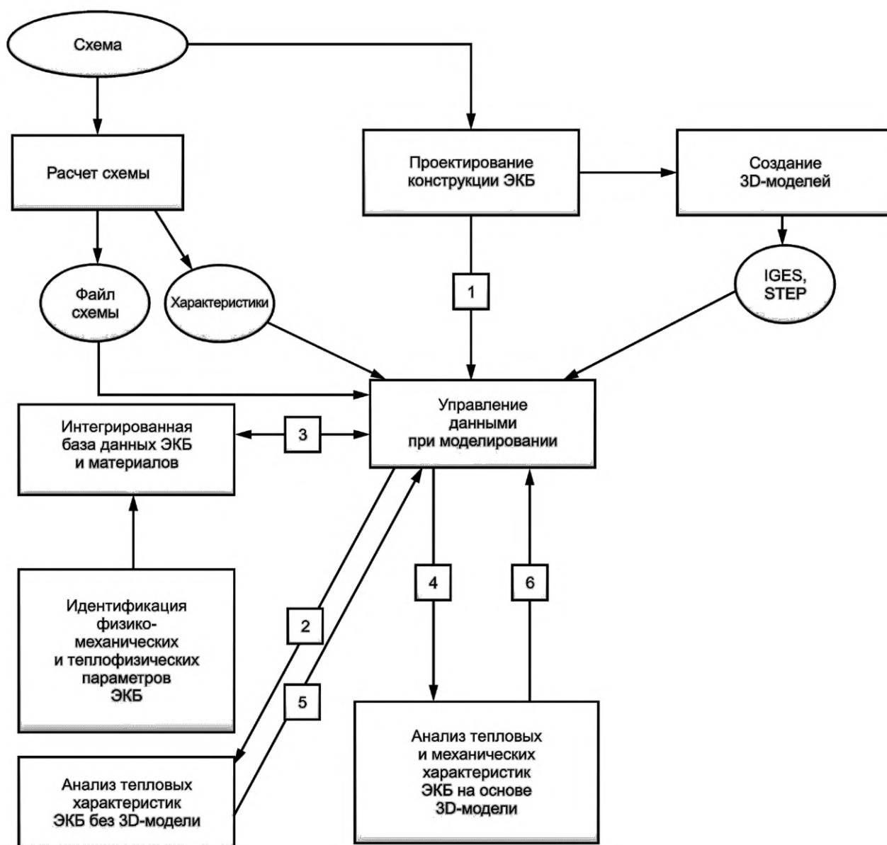
Рисунок 5.1 — Структурная схема САПР ЭКБ
