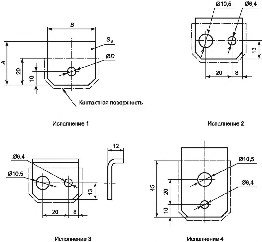
Рисунок 2 — Планки заземления
