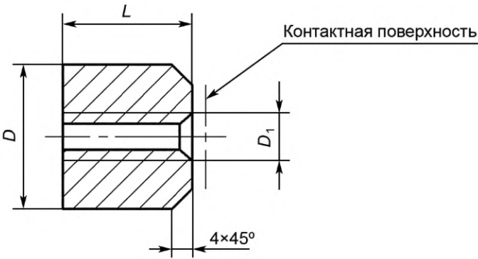
Рисунок 3 — Бонка заземления
