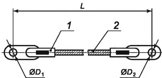
1 — наконечник; 2 — провод
