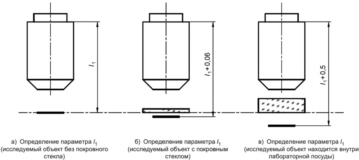
Рисунок А.1 — Примеры определения размеров, относящихся к фокусировке микроскопа и зависящих от толщины покровного стекла
