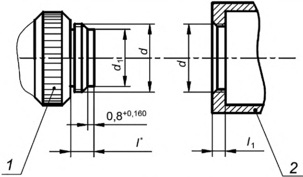
1 — объектив; 2 — тубус
