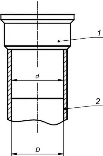
1 — окуляр; 2 — тубус
