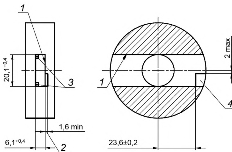
1 — базовая поверхность; 2 — глубина ориентирующей выемки; 3 — контактные пружины; 4 — ориентирующая поверхность
