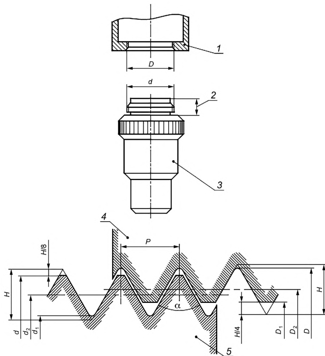
1 — тубус и револьверная головка, с которой соединены объектив и другие элементы микроскопа; 2 — выступающая часть резьбы; 3 — объектив; 4 — внутренняя резьба; 5 — наружная резьба
