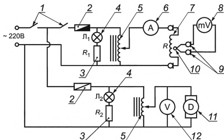
Рисунок 2 — Электросхема центрифуги
