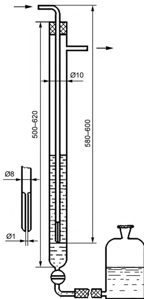
Рисунок 2 — Мононат жидкостный
