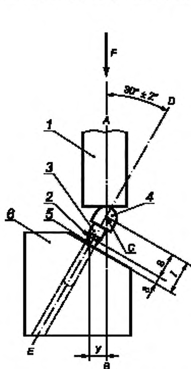
1 — устройство для прикладывания нагрузки [позволяющее осуществлять свободное движение перпендикулярно к направлению нагрузки (см. 5.2.6)]; 2 — номинальный уровень кости (см. 5.3.2); 3 — соединительный компонент; 4 — полусферический нагружаемый элемент; 5 — тело стоматологического имплантата; 6 — держатель образца
