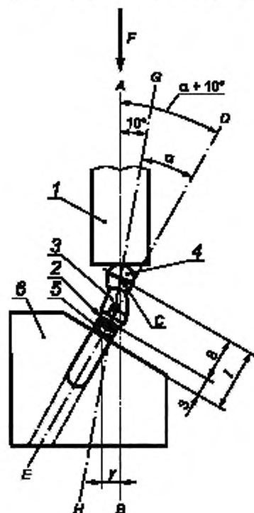
1 — устройство для прикладывания нагрузки [позволяющее осуществлять свободное движение перпендикулярно к направлению нагрузки (см. 5.2.6)]; 2 — номинальный уровень кости (см. 5.3.2); 3 — соединительный компонент; 4 — полусферический элемент нагрузки; 5 — тело стоматологического имплантата; 6 — держатель образца
