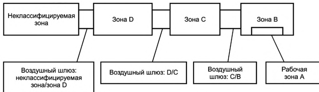
Рисунок F.2 — Обычное чистое помещение
