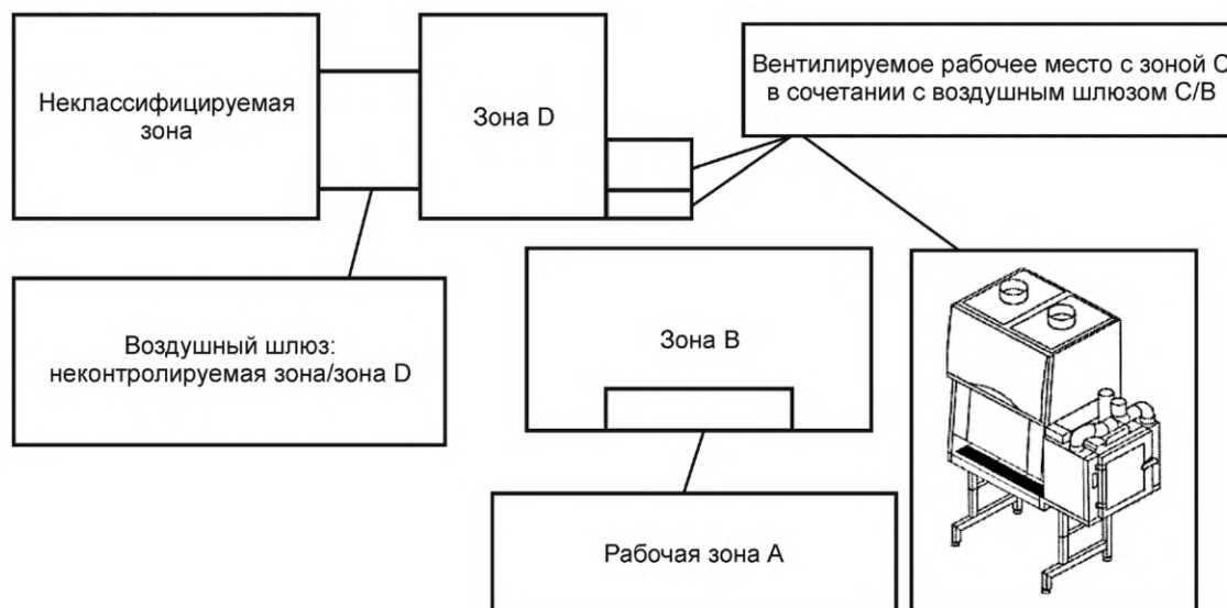
Рисунок F.1 — Вентилируемый бокс класса С в сочетании с воздушными шлюзами
