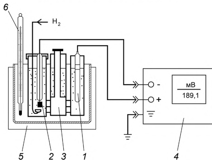
Схема установки для определения потенциала эталонного электрода сравнения E_{эТ}
