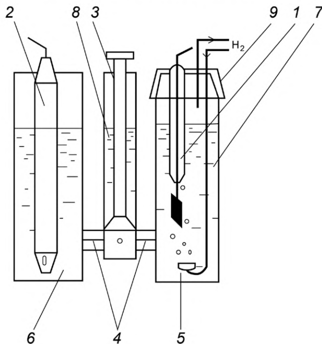
Схема электрохимической ячейки для определения потенциала эталонного электрода сравнения E_{\text{эт}}
