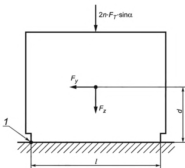
1 — ребро опрокидывания
