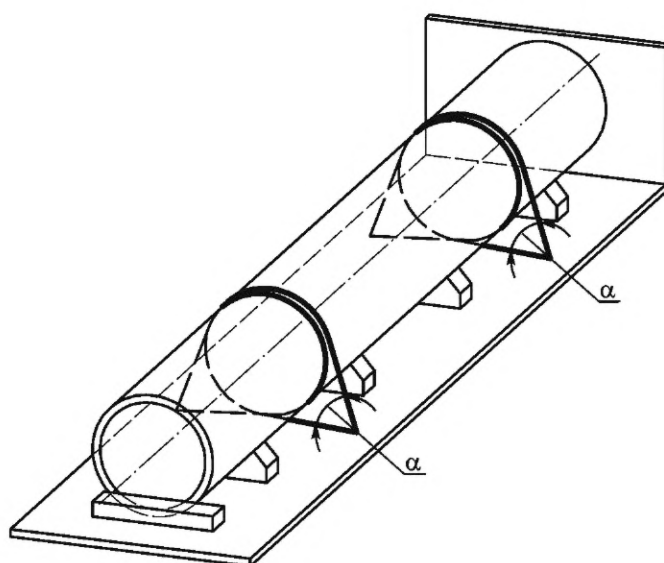
Рисунок 11 — Крепление петель
