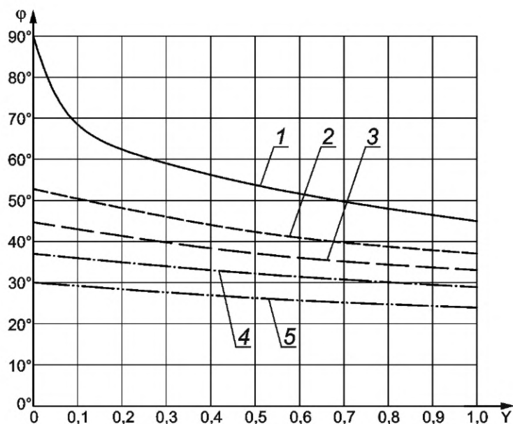
Рисунок 18 — Диаграмма для определения значения угла наклона грузовой платформы \varphi
