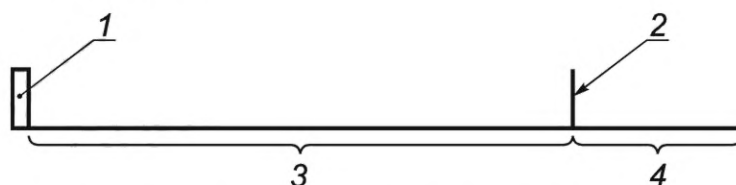
1 — начальная точка испытательного заезда и искусственная неровность высотой от 10 до 20 мм и шириной примерно 500 мм под углом от 60^\circ до 80^\circ ; 2 — стационарное дополнительное устройство замедления; 3 — участок ускорения для достижения скорости от 35 до 40 км/ч; 4 — участок полной остановки
