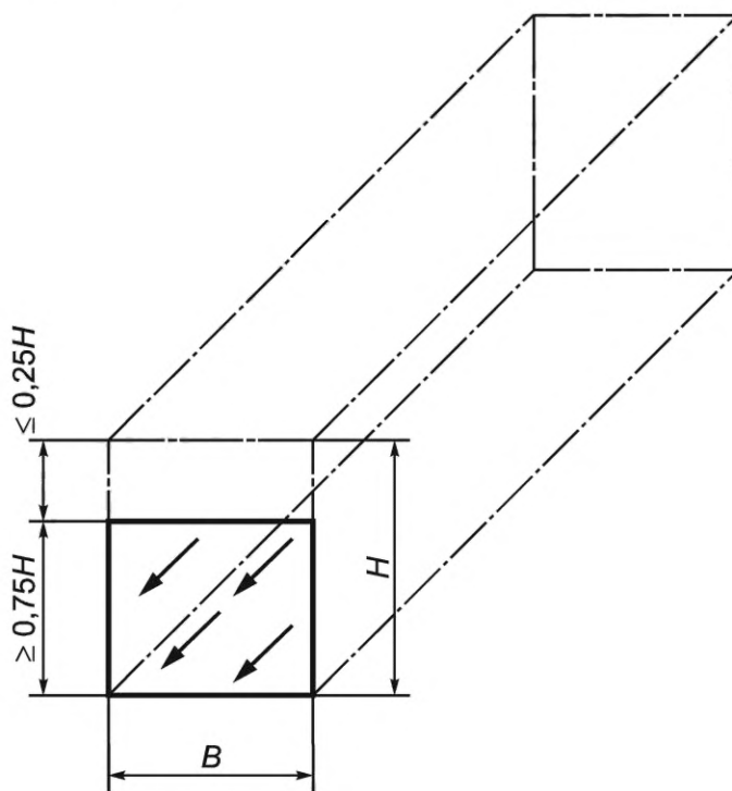
Рисунок 2 — Приложение испытательной нагрузки при испытаниях передней стенки кузова
