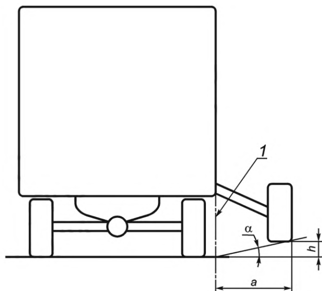
1 — перпендикуляр; a — расстояние между внешним габаритом прицепа и внешней вертикальной линией вспомогательного колеса в мм; h — высота нижней точки вспомогательного колеса над уровнем грунта, мм; \alpha — минимальный угол в зависимости от значений a и h ( \text{tg } \alpha = h/a )
