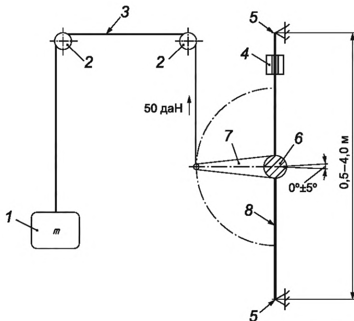
1 — груз; 2 — направляющий шкив; 3 — веревка; 4 — датчик измерения силы или динамометр; 5 — точка закрепления ремня; 6 — ось с прорезью; 7 — рукоять натяжного устройства; 8 — лента ремня
