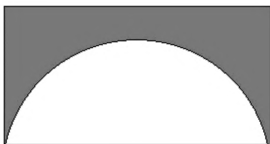
Рисунок 7 — Место отбора пробы для анализа поглощения в поперечных сечениях пиломатериалов и брусьев, когда требуется сплошная пропитка заболони (а) или сплошная пропитка заболони и определенное проникновение в ядро (б)
