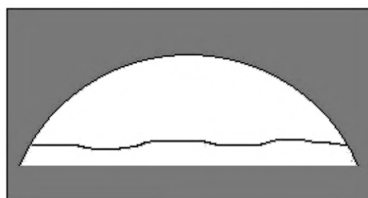
Рисунок 7 — Место отбора пробы для анализа поглощения в поперечных сечениях пиломатериалов и брусьев, когда требуется сплошная пропитка заболони (а) или сплошная пропитка заболони и определенное проникновение в ядро (б)
